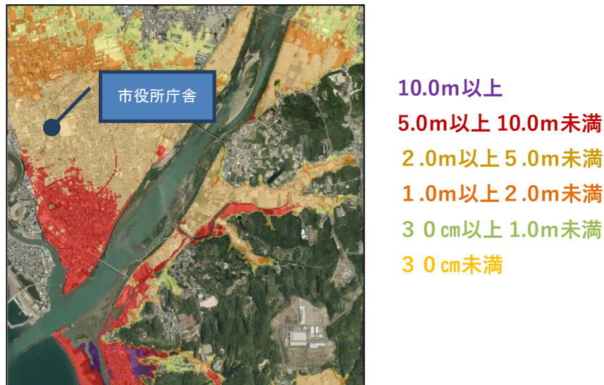
◆図：南海トラフ巨大地震による浸水予想図
