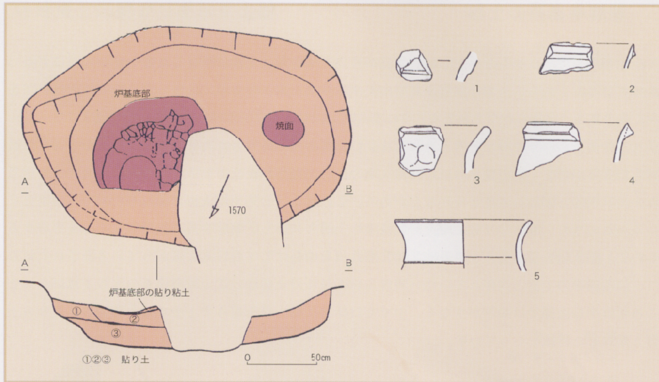
溶炉遺構と時期を示す土器 溶炉遺構(1～4)・土杭1570(5)
