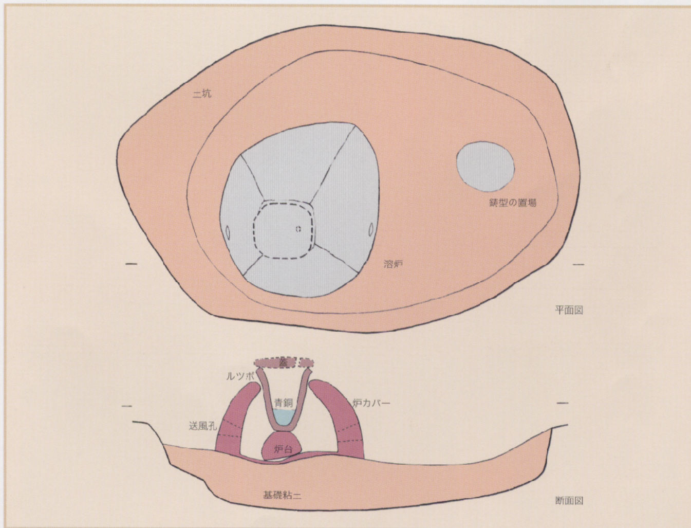
溶炉遺構の復元図
