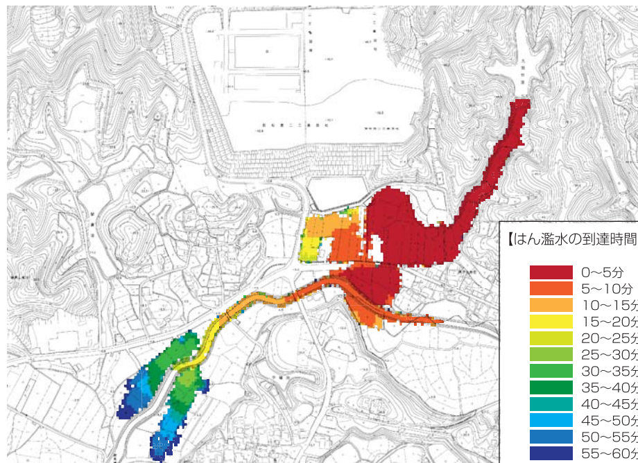
はん濫水到達時間 【九田谷池】
